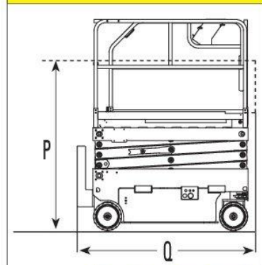
Macchina chiusa con ringhiera abbassate Stowed machine with folded-down rails
